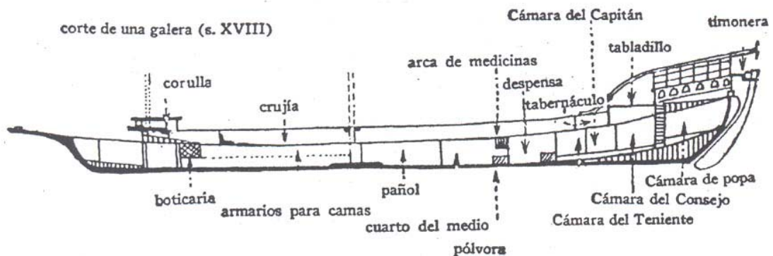
Corte de una galera capitana de la primera mitad del siglo XVIII. Dibujo del almirante Guillén según lámina del álbum del Marqués de la Victoria.
